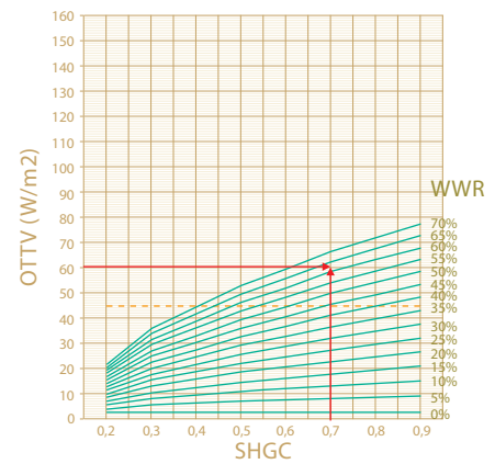
WWR Dinding Selatan (180°)
