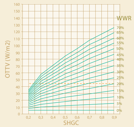
WWR Dinding Tenggara (135°)
