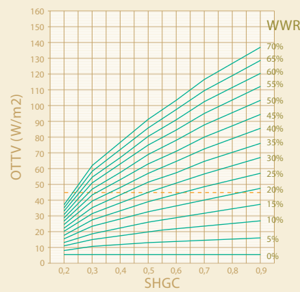
WWR Dinding Selatan (180°)
