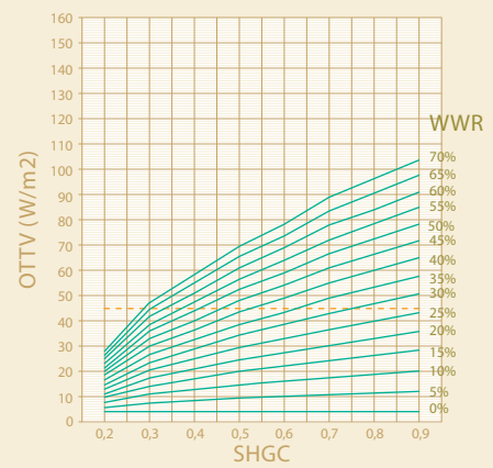
WWR Dinding Barat Daya (225°)
