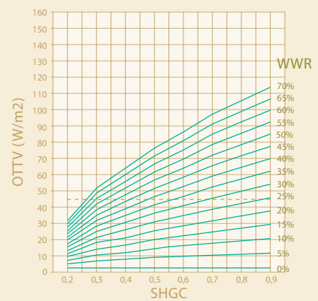
WWR Dinding Barat Laut (315°)
