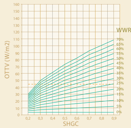
WWR Dinding Timur (90°)
