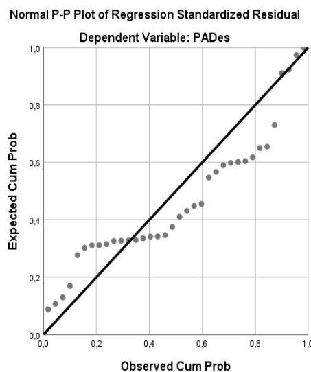
Grafik 2 Normal P-Plot
