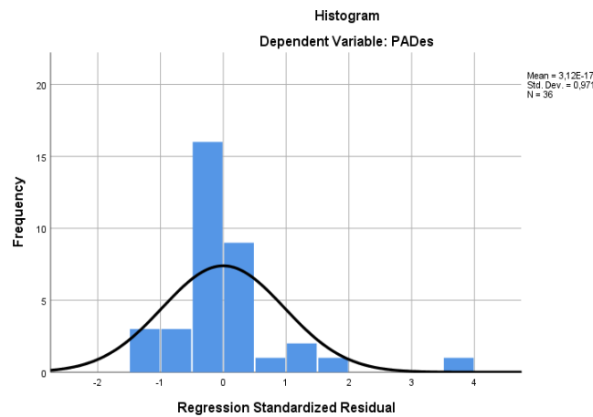
Grafik 1 Histogram
